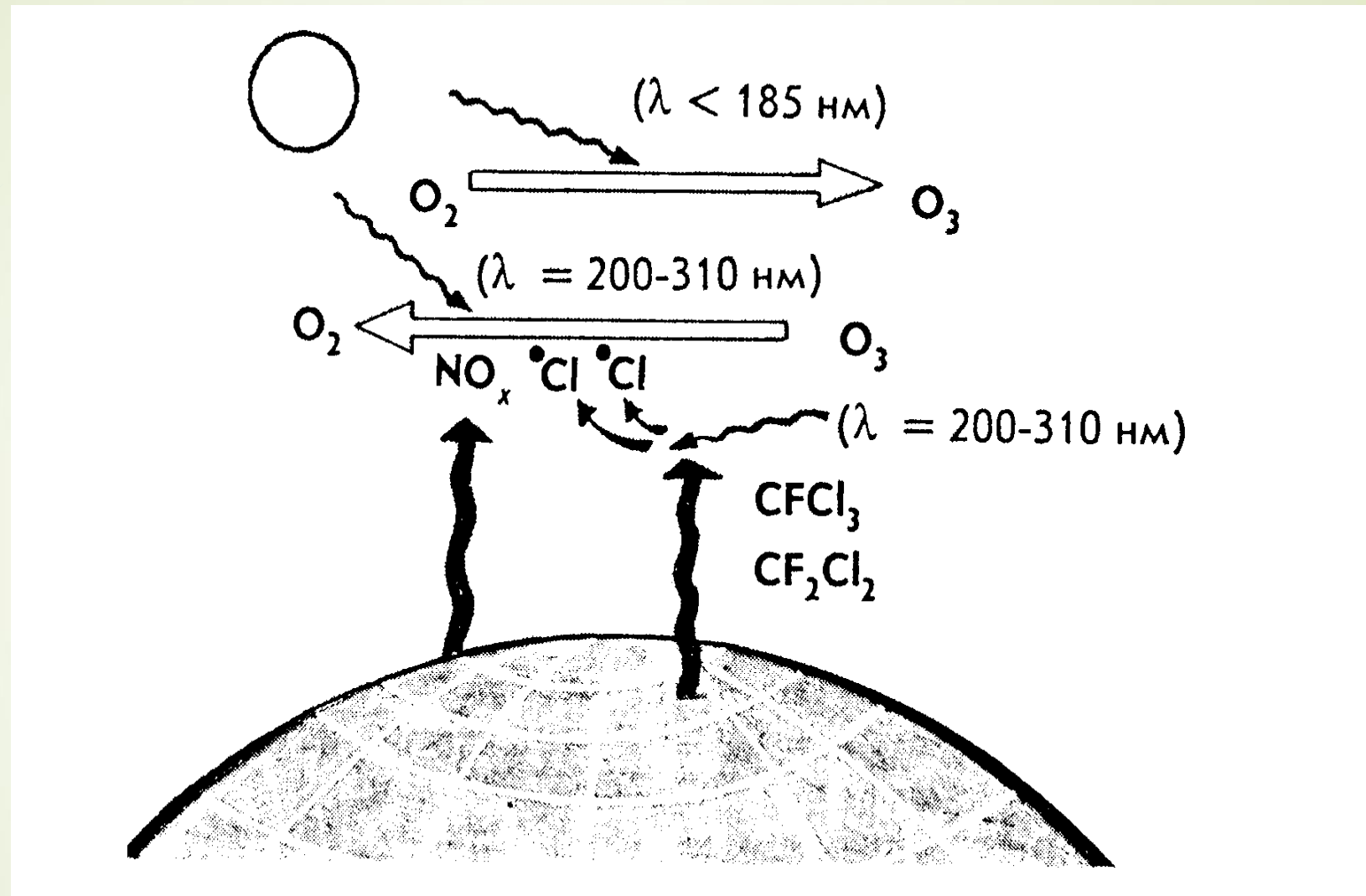
Рис. 9. Схема впливу флуорохлоровуглеводнів та нітроген оксидів на озоновий шар.
